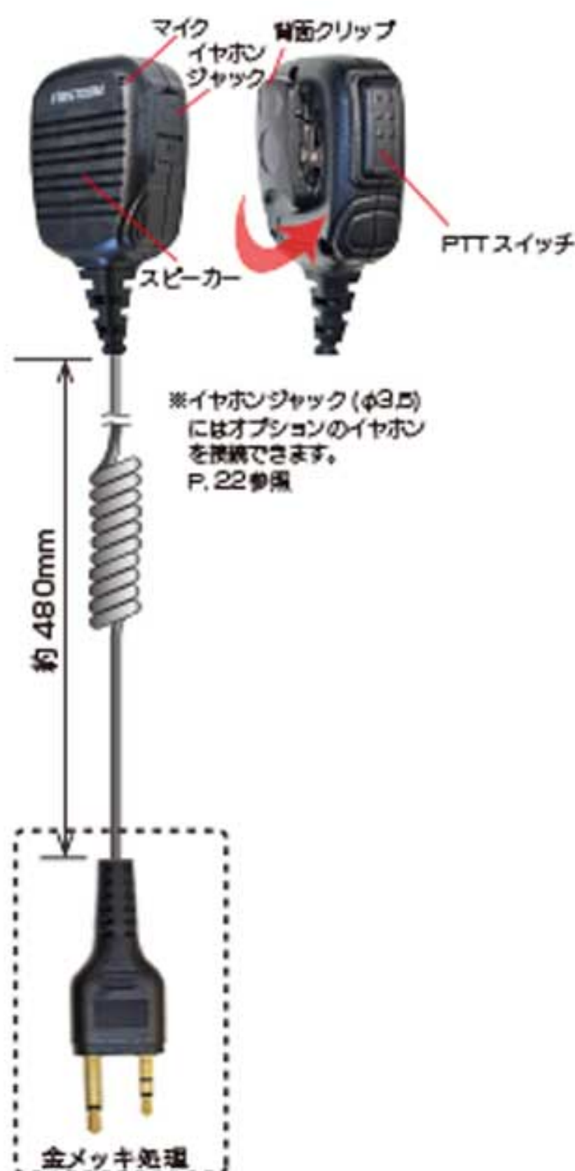
接続プラグタイプ別参照
