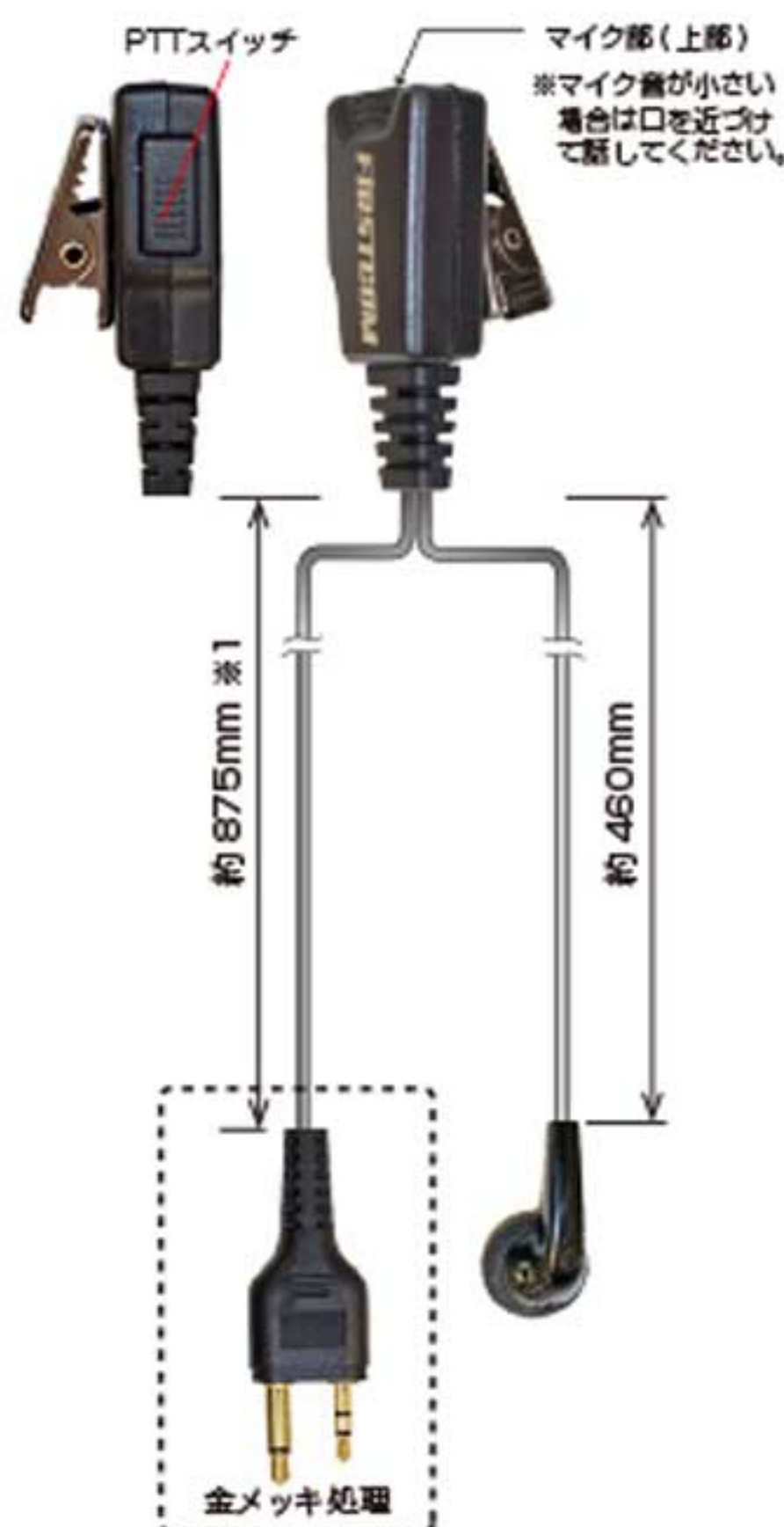
接続プラグタイプ別参照
