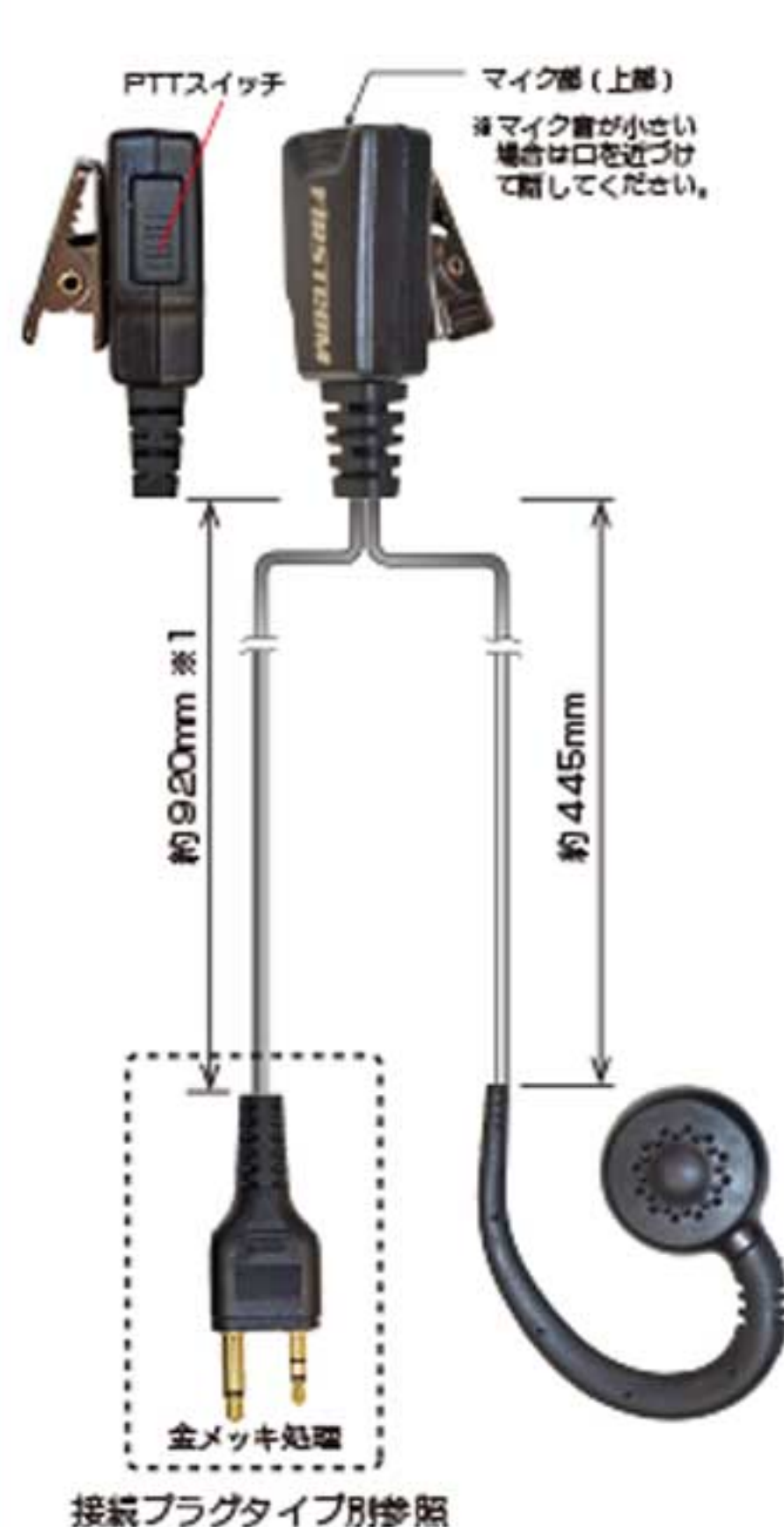
WPタイプ (ALINCO/YAESU/FRC 対応)
