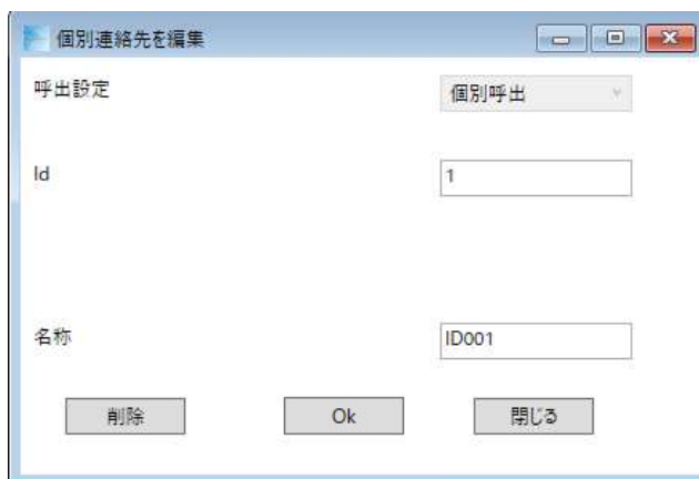
個別呼出ウィンドウ中の 1～1000 のリストをダブルクリックすると、個別連絡先を編集・ウィンドウが表示されます。Id の設定範囲は 1～65519 です。名称の入力可能文字数は、全角 8 文字以下、半角英数字 16 文字以下となります。
