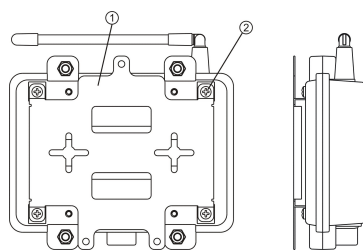
「背面図」壁面取付け金具
